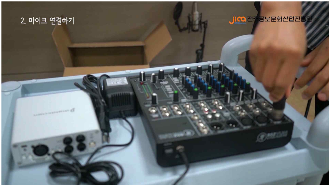
믹서 연결 (마이크 두 대 연결)
